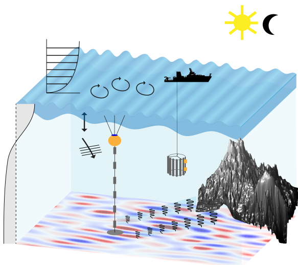
Schematische Darstellung der Gezeitenwellen südlich der Azoren (rot/blau), der Austauschprozesse, und unserer Messgeräte CTD/LADCP Sonde (am Schiff) und einer verankerten Messkette zur Beobachtung von zeitlichen Schwankungen.
